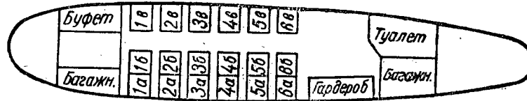
ИЛ-14
