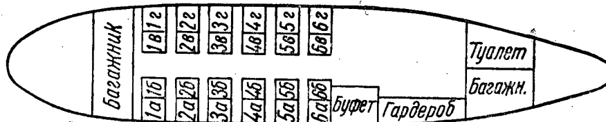
ИЛ-14М
