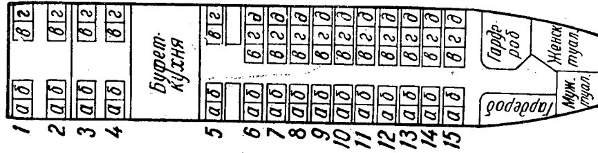
ТУ-104А
